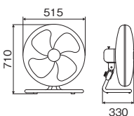
【寸法図】(単位:mm)
