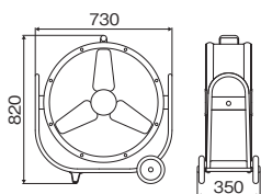
【寸法図】(単位:mm)
