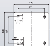
壁面設置金具(穴寸法図)
