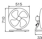
【寸法図】(単位:mm)
