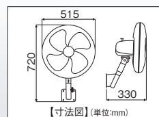
【寸法図】(単位:mm)
