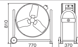
【寸法図】(単位:mm)
