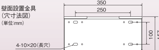
【寸法図】(単位:mm)
