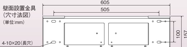
【寸法図】(単位:mm)
