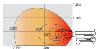
【温度分布図(周囲温度0℃)】
