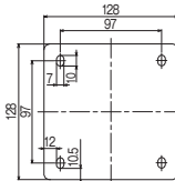
壁面設置金具 (穴寸法図)
