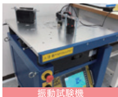
振動試験機
