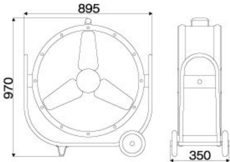
【寸法図】(単位:mm)
