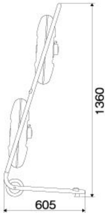
【寸法図】(単位:mm)
